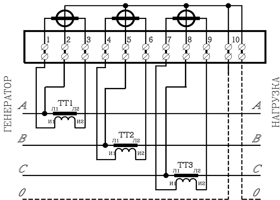
Типовая схема подключения трехфазного электросчетчика с помощью трех трансформаторов тока и трех трансформаторов напряжения к трехфазной 3-х или 4-х проводной сети
