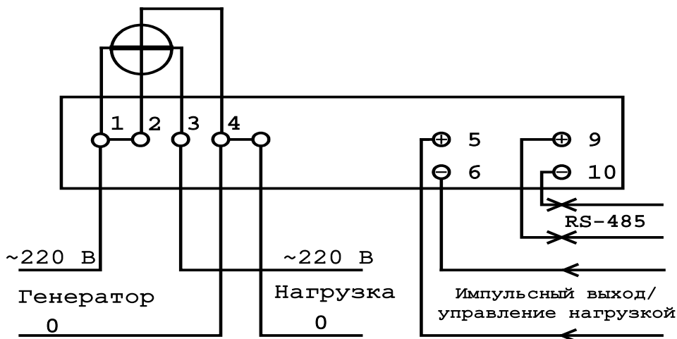
Типовая схема подключения трехфазного электросчетчика к трехфазной 3-х или 4-х проводной сети
